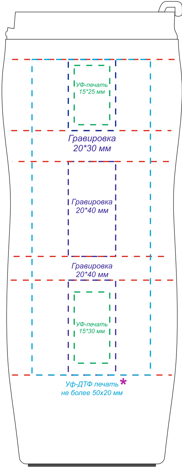
Вид справа
