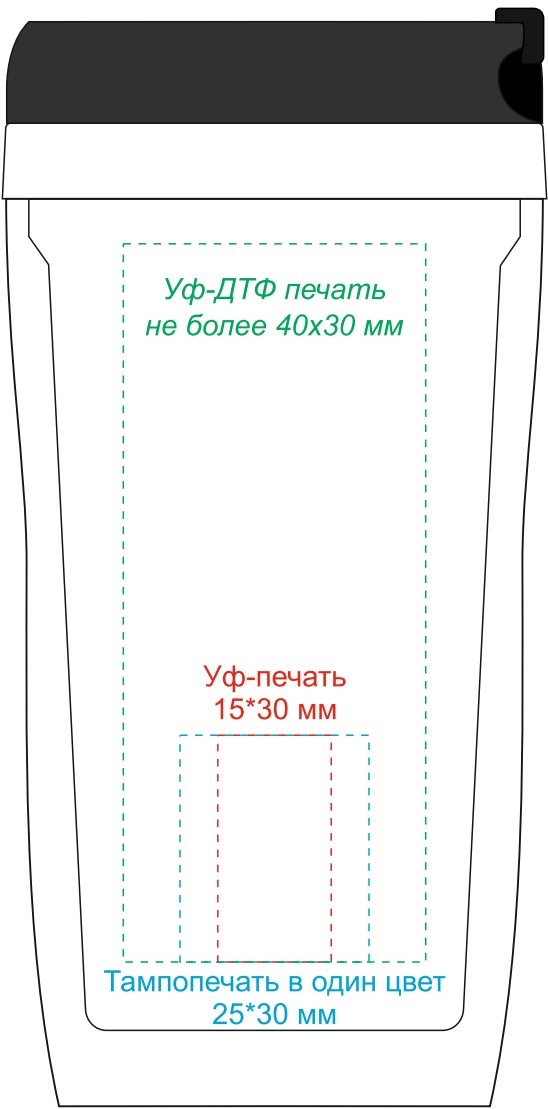
Вид слева
