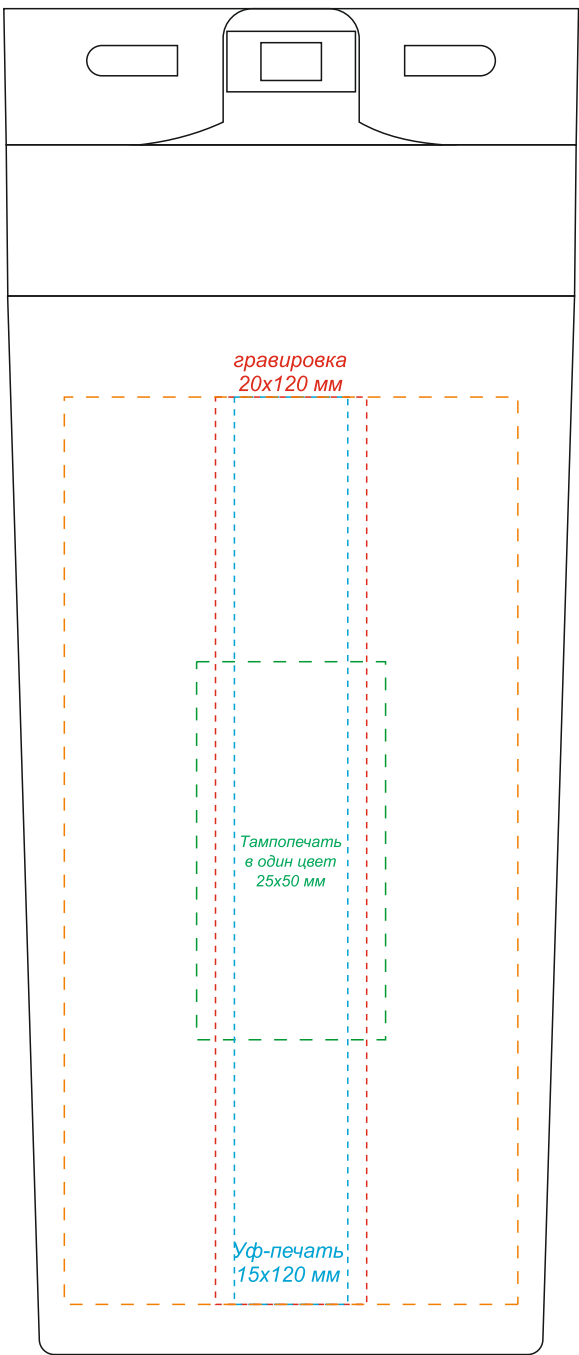
вид сзади
