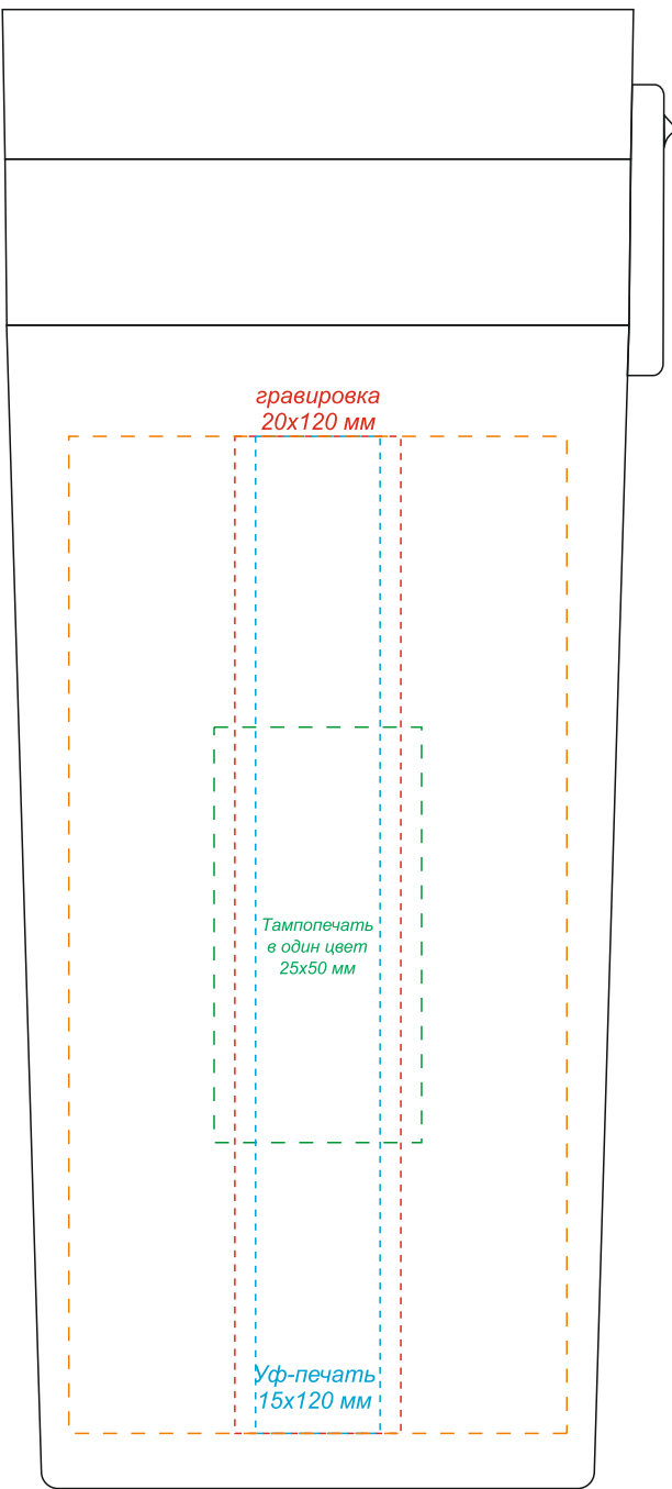
вид слева
