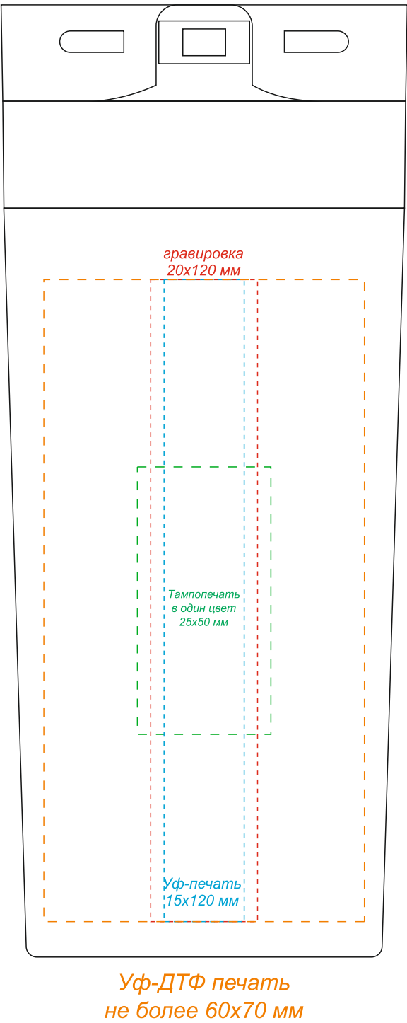
вид сзади
