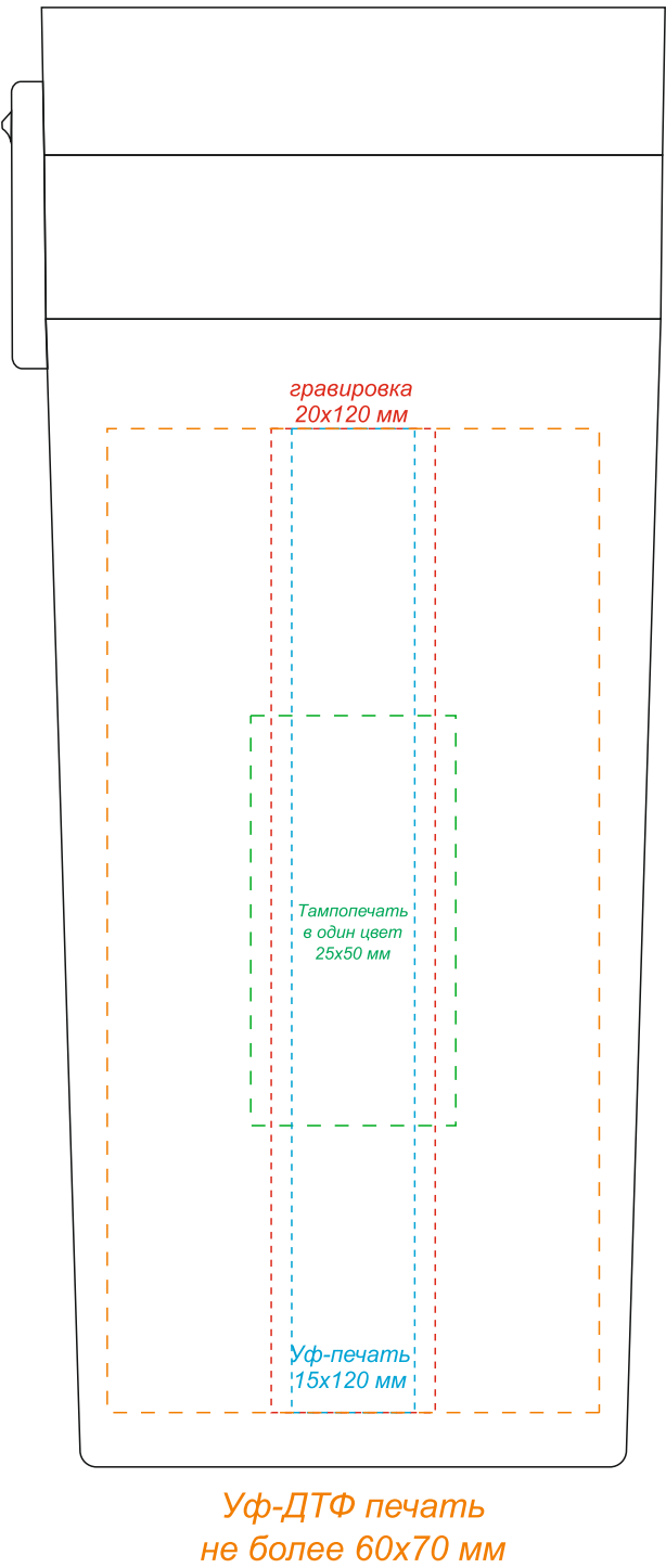
вид справа
