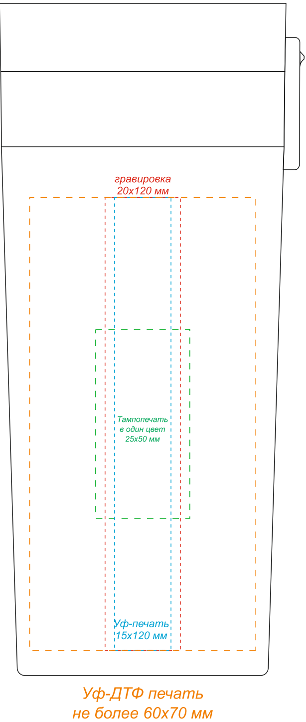
вид слева
