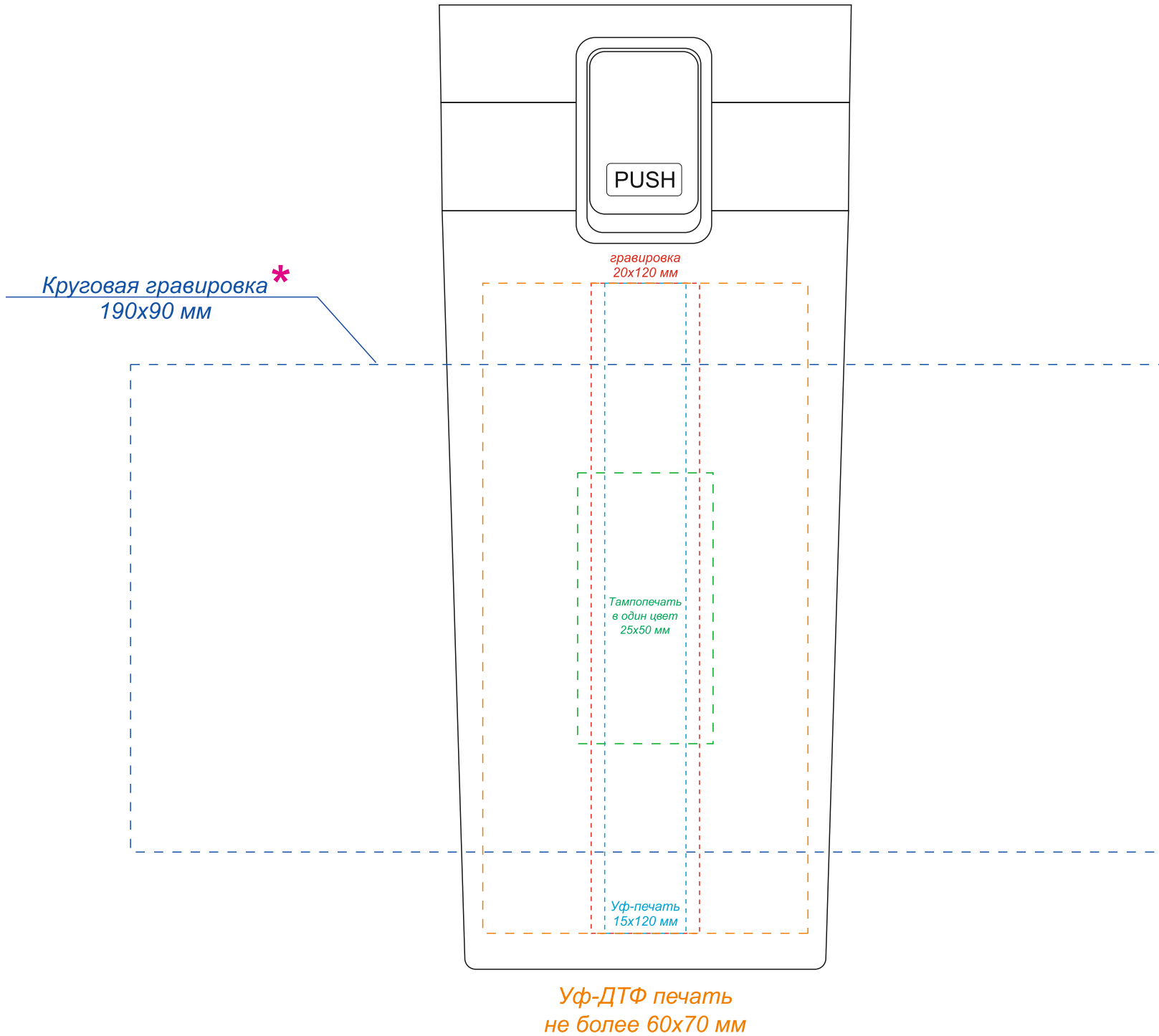
вид спереди
