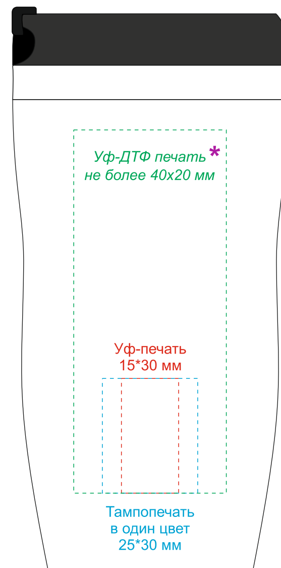
Вид справа
