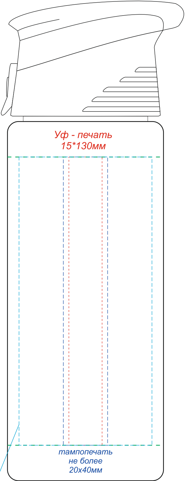
вид справа
