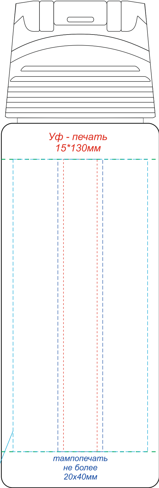
вид сзади
