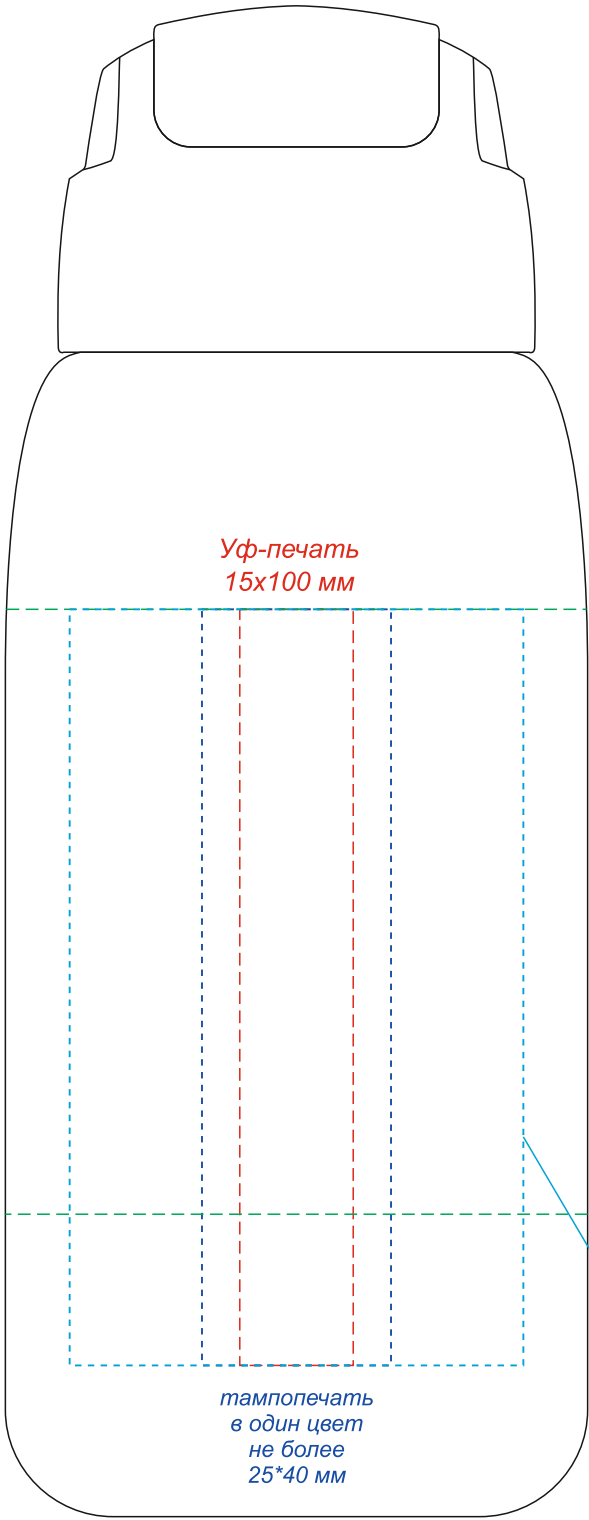
вид спереди
