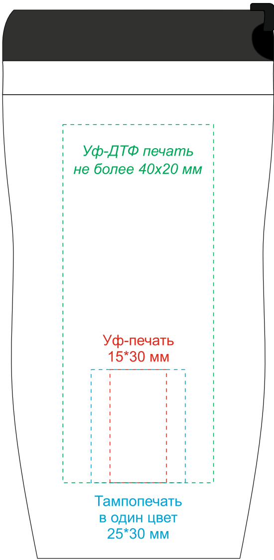
Вид слева
