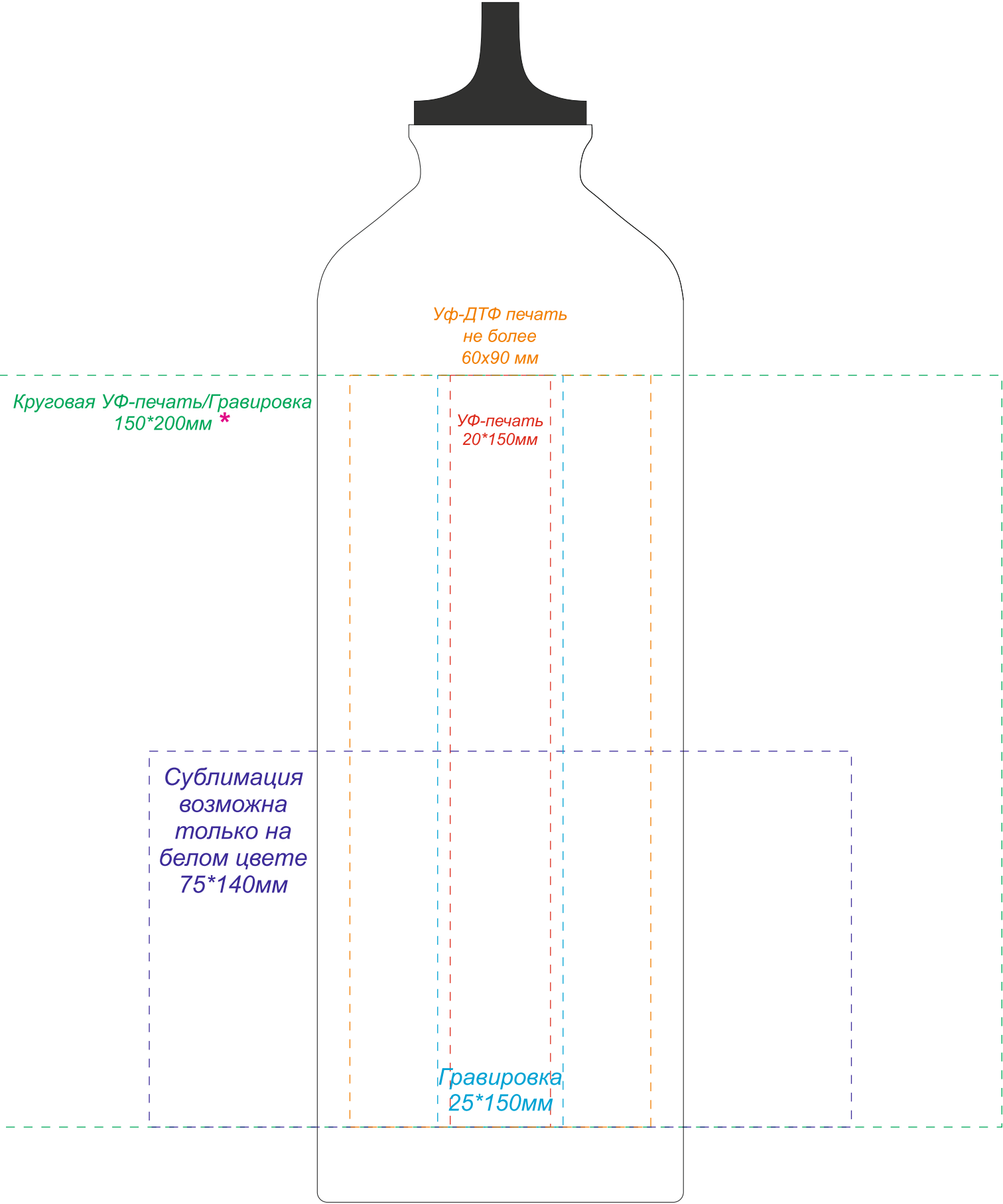
спереди
