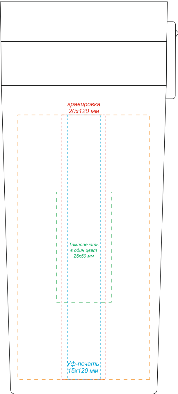
вид слева
