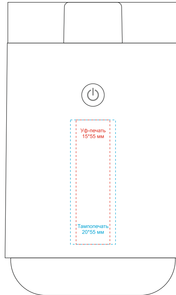
Вид спереди
